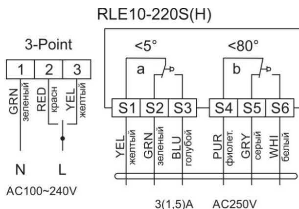
Рисунок 6.2 - Схема (P-Ik/220)
