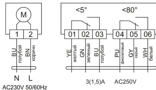
Рисунок 6.12 - Схема (M-IIIk/220)
