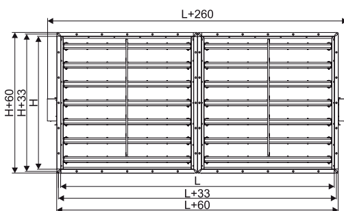
Рисунок 2.5 - Кассетное исполнение - 2и
