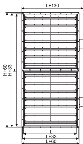
Рисунок 2.3 - Кассетное исполнение - 1и
