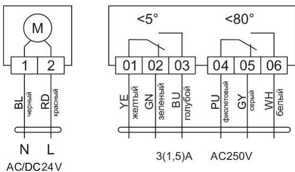
Рисунок 6.11 - Схема (M-IIIk/24)
