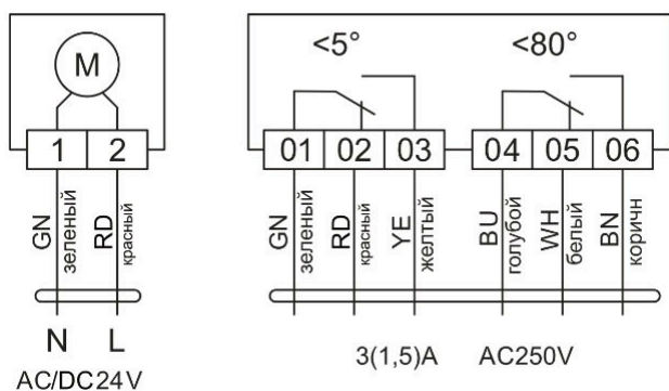
Рисунок 6.9 - Схема (M-IIk/24)
