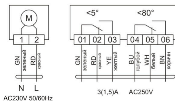
Рисунок 6.10 - Схема (M-IIk/220)
