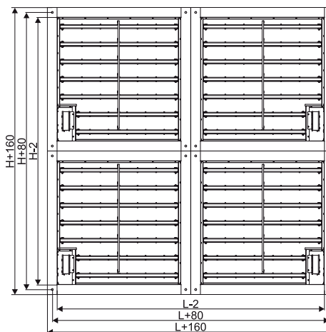
Рисунок 2.7 - Кассетное исполнение - 3и
