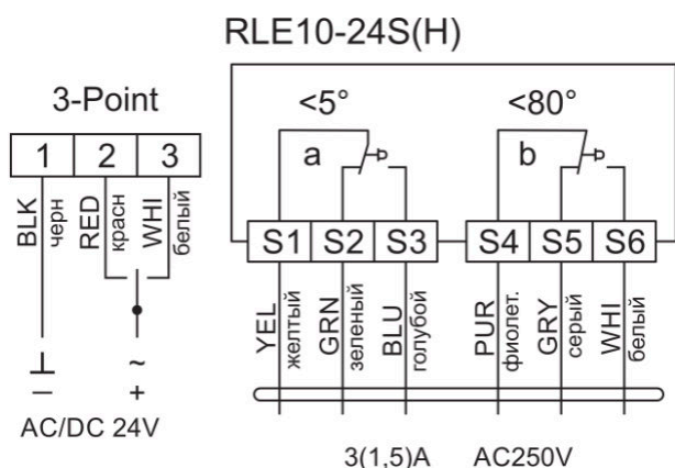
Рисунок 6.1 - Схема (P-Ik/24)
