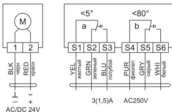
Рисунок 6.7 - Схема (M-Ik/24)
