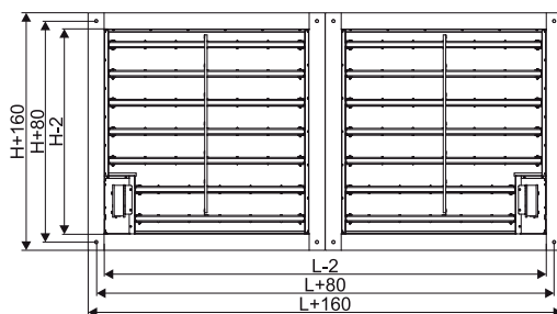
Рисунок 2.8 - Кассетное исполнение - 2и
