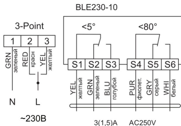
Рисунок 6.6 - Схема (P-IIIk/220)
