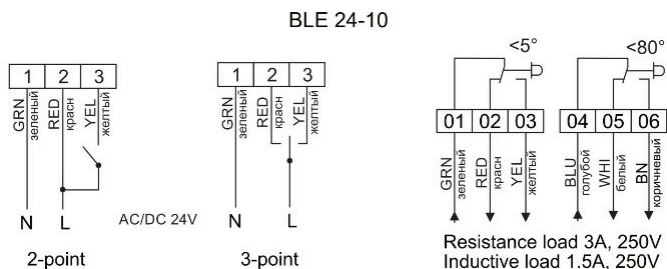
Рисунок 6.1 - Схема (P-Ik/24)
