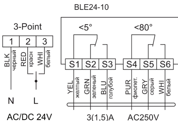
Рисунок 6.5 - Схема (P-IIIk/24)
