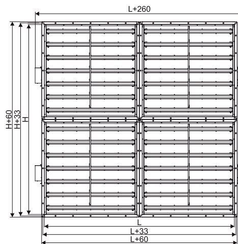
Рисунок 2.4 - Кассетное исполнение - 3и
