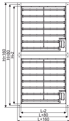
Рисунок 2.6 - Кассетное исполнение - 1и
